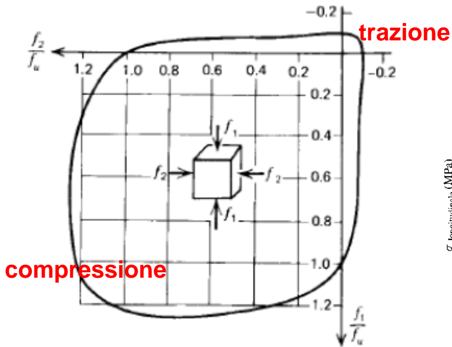
Legame costitutivo bi-assiale
