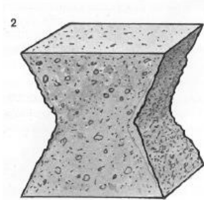
Forma a doppia piramide dopo la prova di compressione
